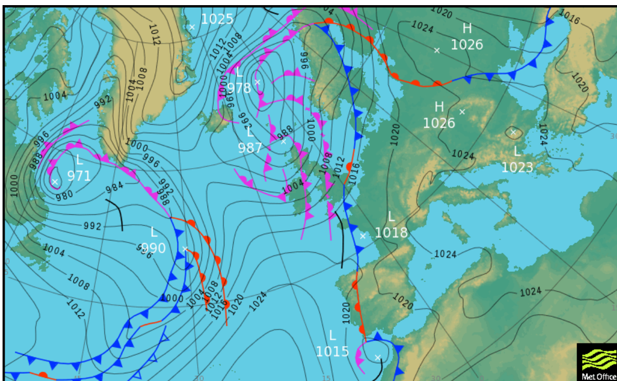
Situation synoptique prévue pour Lundi 18 Février 2019 à 12H00 UTC (Source : Service météorologique britannique)
