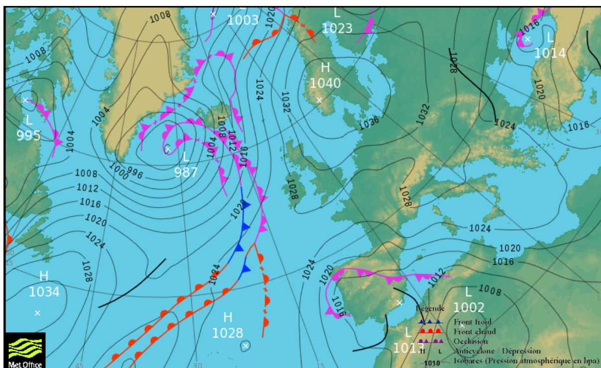
Situation synoptique prévue pour le Samedi 20 Avril à 12H00 UTC (Source : Service météorologique britannique)
