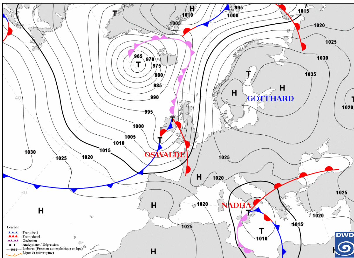
Situation synoptique prévue pour Samedi 15 Décembre 2018 à 12H00 UTC (Source : Deutscher Wetterdienst)
