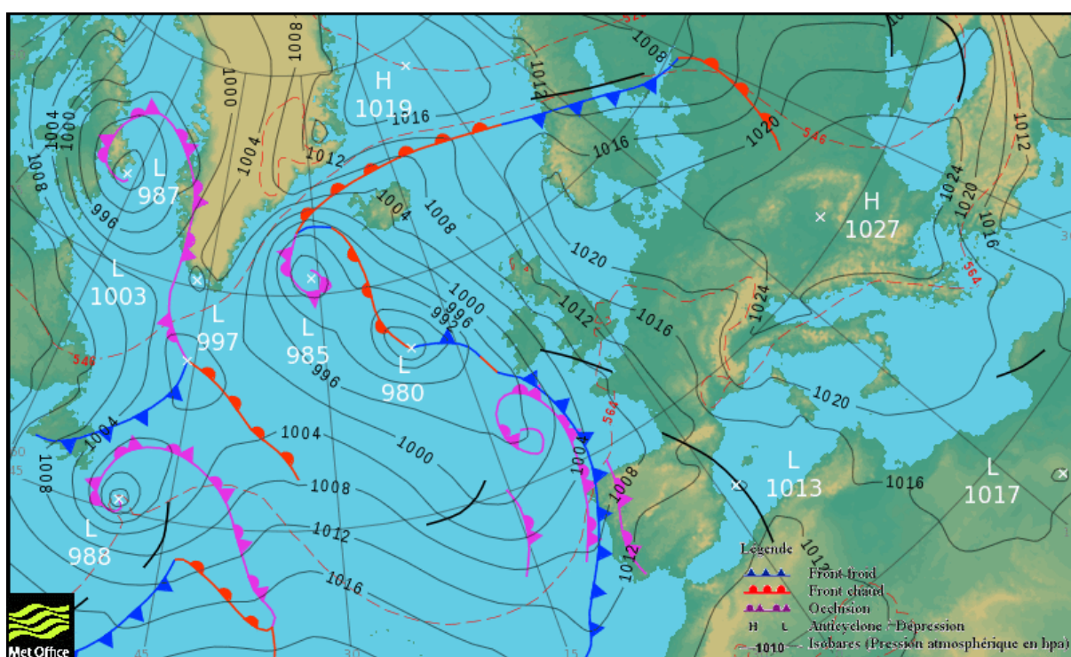
Situation synoptique prévue pour le Samedi 21 Septembre à 12H00 UTC (Source : Service météorologique britannique)
