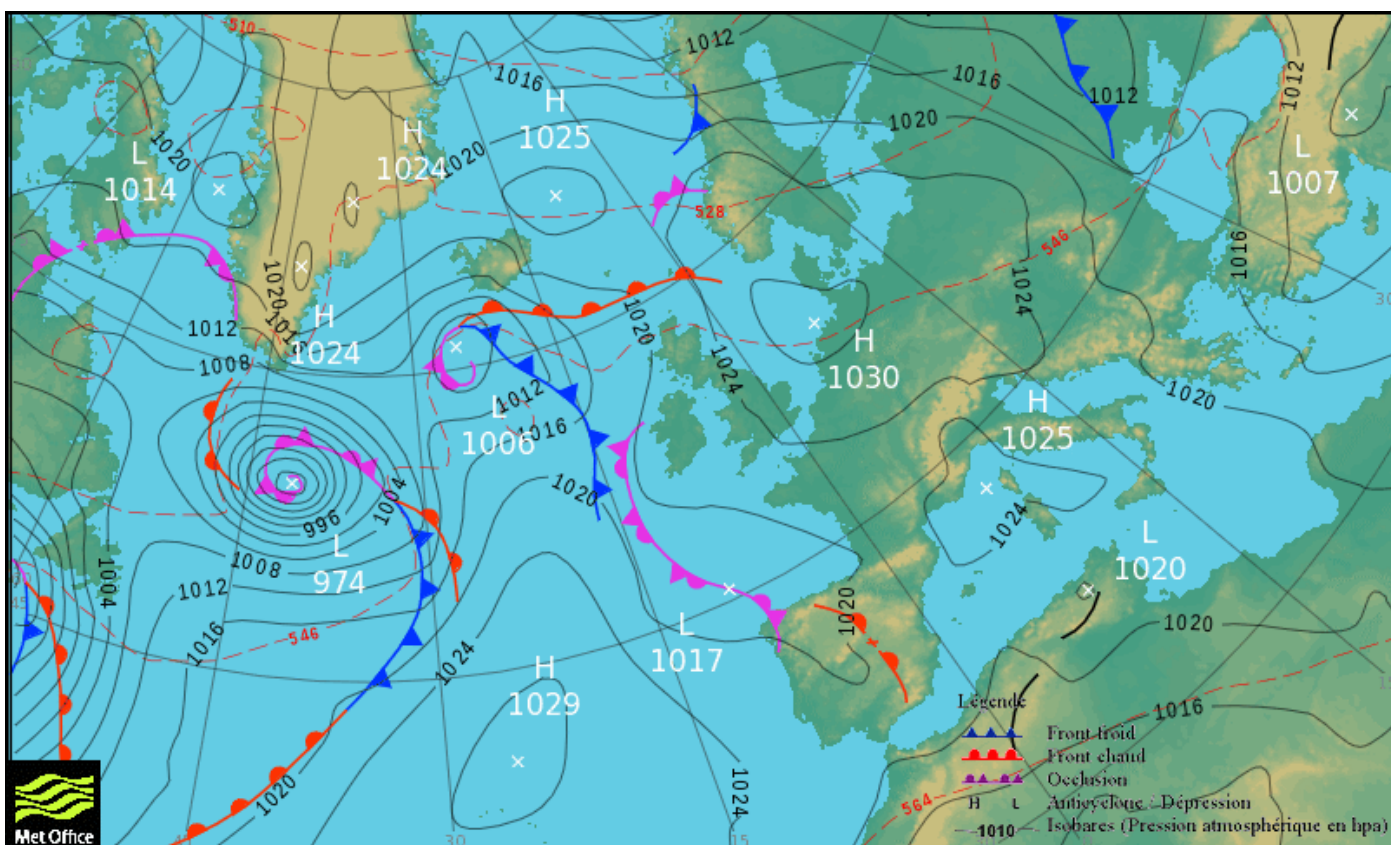
Situation synoptique prévue pour le Vendredi 10 Avril 2020 à 12H00 UTC (Source : Service météorologique britannique)
